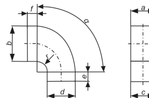
21 BA / Bogenübergang
