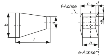
41 UA / Übergang, asymmetrisch
