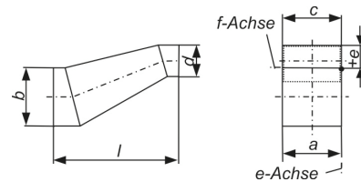
61 EA / Etagenübergang
