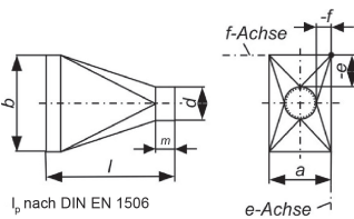
50 RS / Rohrübergang, symmetrisch
