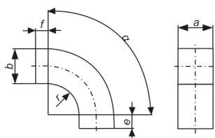
20 BS / Bogen, symmetrisch
