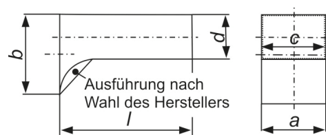
15 SU / Übergangsstutzen
