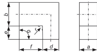
41 UA / Übergang, asymmetrisch
