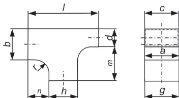
70 TG / T-Stück, oben gerade
