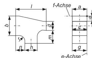
71 TA / T-Stück, oben schräg
