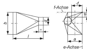
51 RA / Rohrübergang, asymmetrisch
