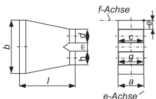
80 HS / Hosenstück
