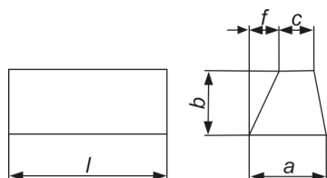
14 TL / Luftleitung in Trapezform
