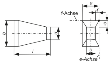
40 US / Übergang, symmetrisch
